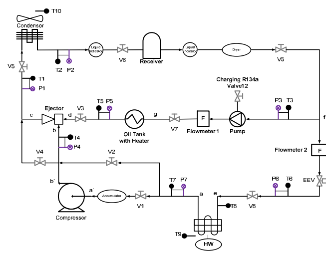
汽车废热驱动空调原理图
