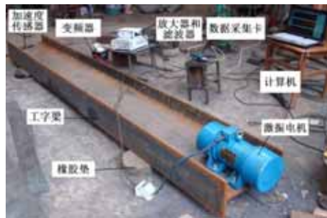
振动时效装置
