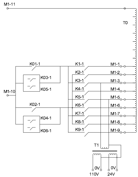
10kV 新型有载分接开关主接线图
