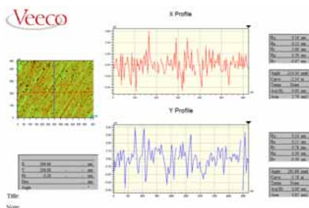
45 钢镍基抛光表面在白光干涉仪中的抛光结果
