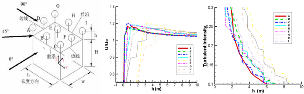
图 2 建筑物顶风机安装参考位置 (a) 各参考位置的风速比 (b) 各参考位置的湍流强度 图 3 平顶建筑物各参考位置的风速比与湍流强度的曲线图 对建筑物两边的风场分析见图 4，(a)、(b)和(c)是在不同的高度平面上的风场，可以为风机的安装选址提供理论根据。
