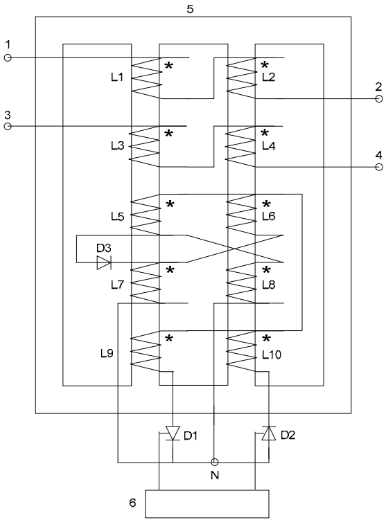
多功能变压器主接线图
