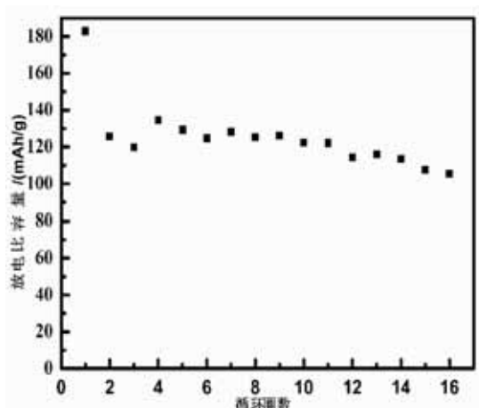
产品 \text{h-LiMnBO}_3@\text{C} 的锂离子电池循环性能图
